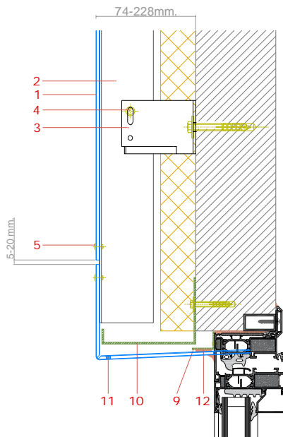
SECÇÃO VERTICAL REMATE JANELA SUPERIOR
