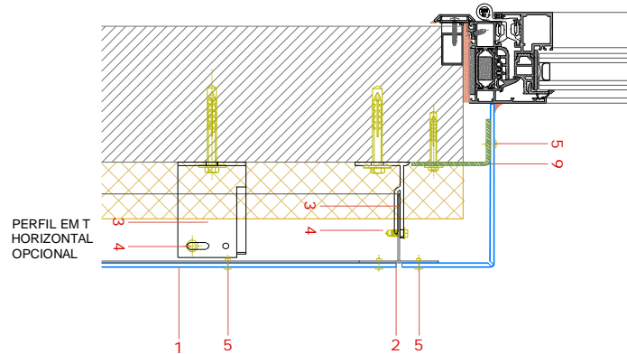
SECÇÃO VERTICAL REMATE JANELA
