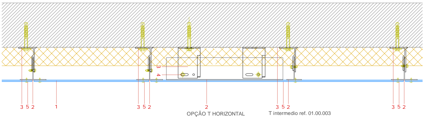
SECÇÃO HORIZONTAL
