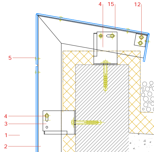
SECÇÃO VERTICAL REMATE DA FACHADA SUPERIOR
